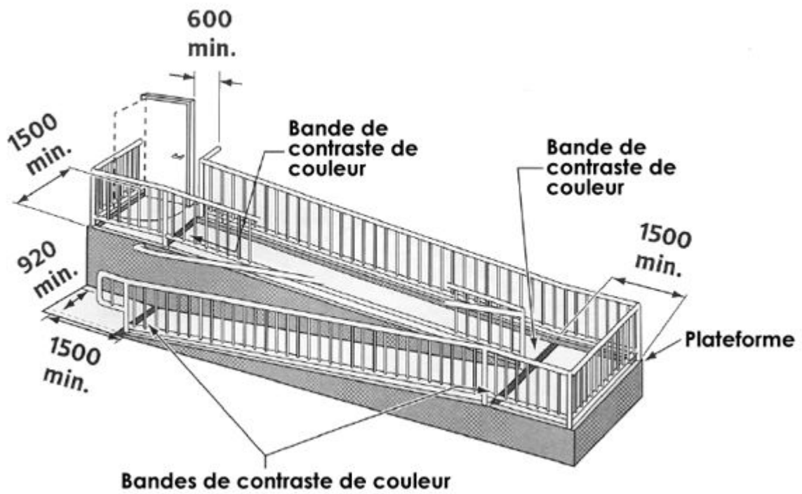
Illustration 3 - Rampes d'accès et plates formes
