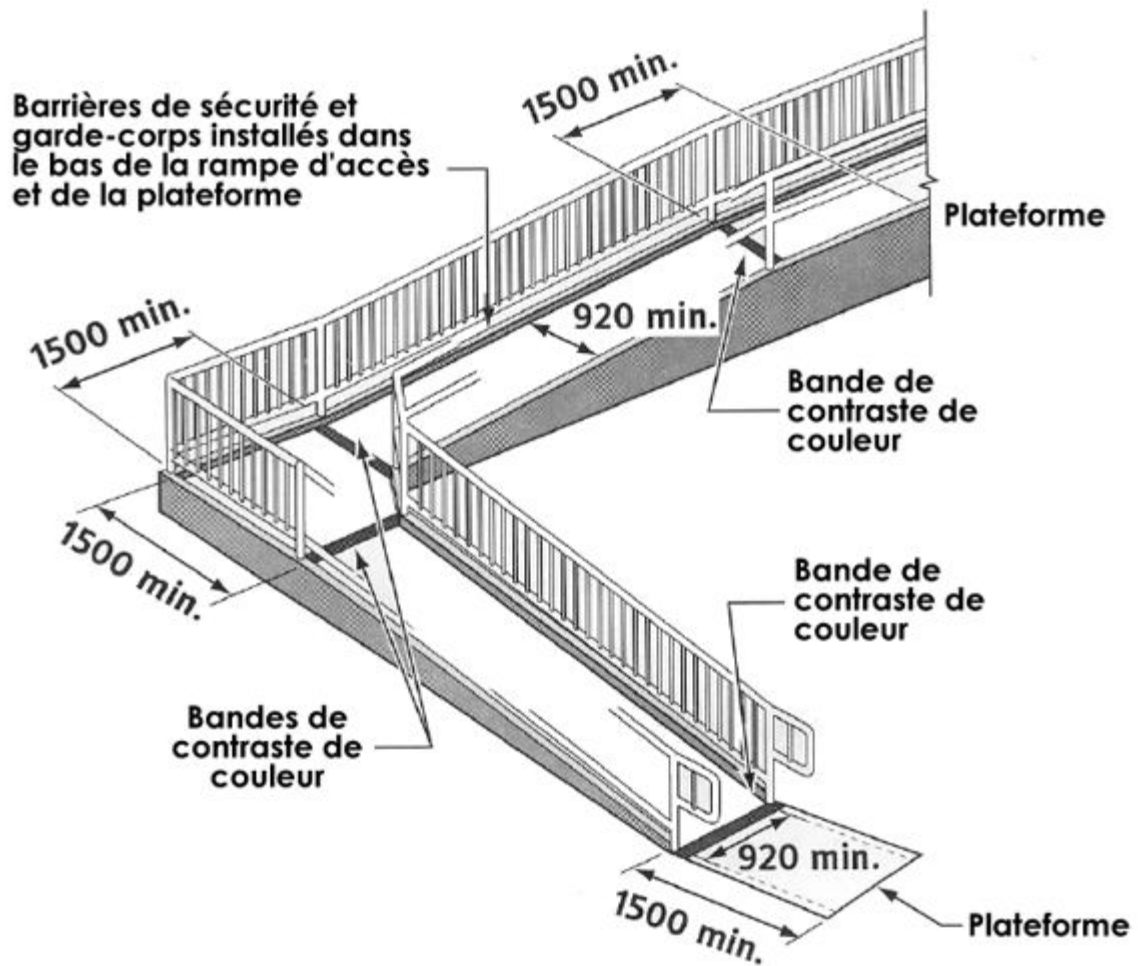
Illustration 2 - Rampes d'accès et plates formes
